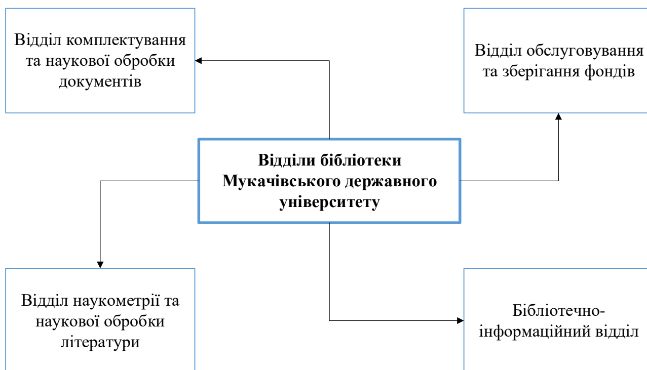
Рис. 2.1. Структура бібліотеки
