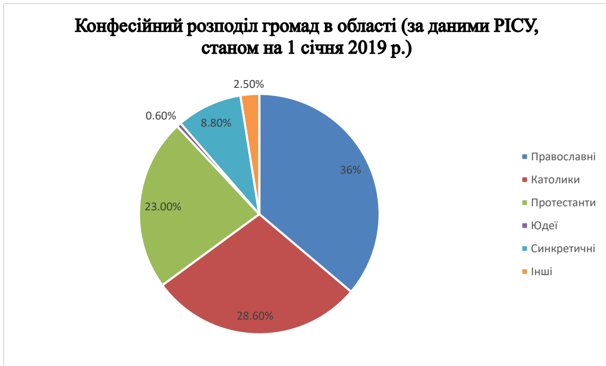
Діаграма 1
