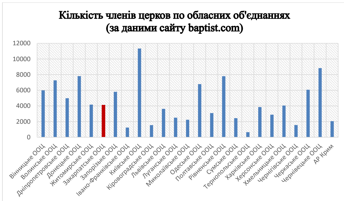
Діаграма 2
