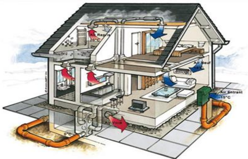
Рис. 5. PAS. Модель пасивного будинку
