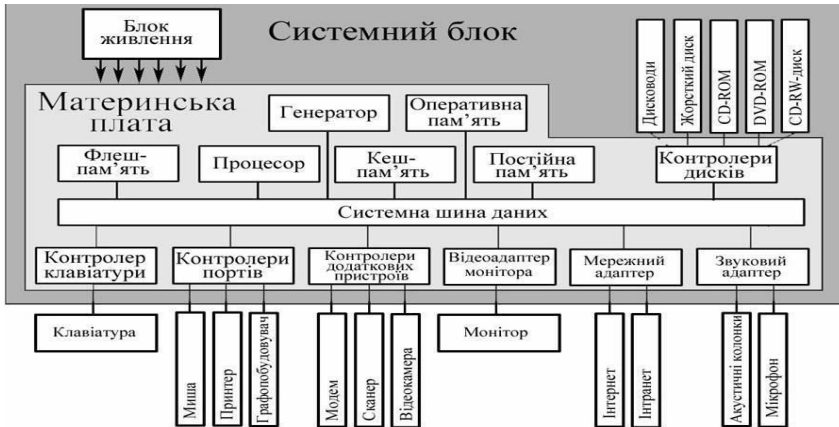
Структурна схема ПК та її складові
